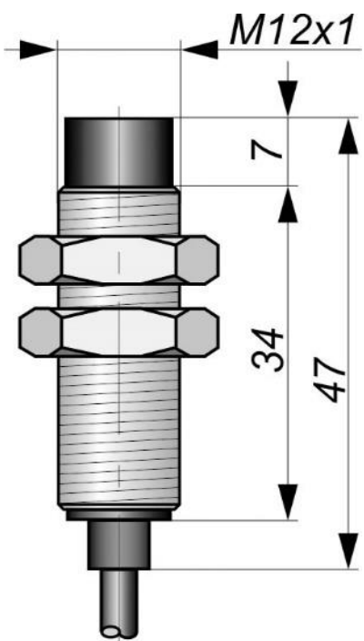
Габаритный чертеж
