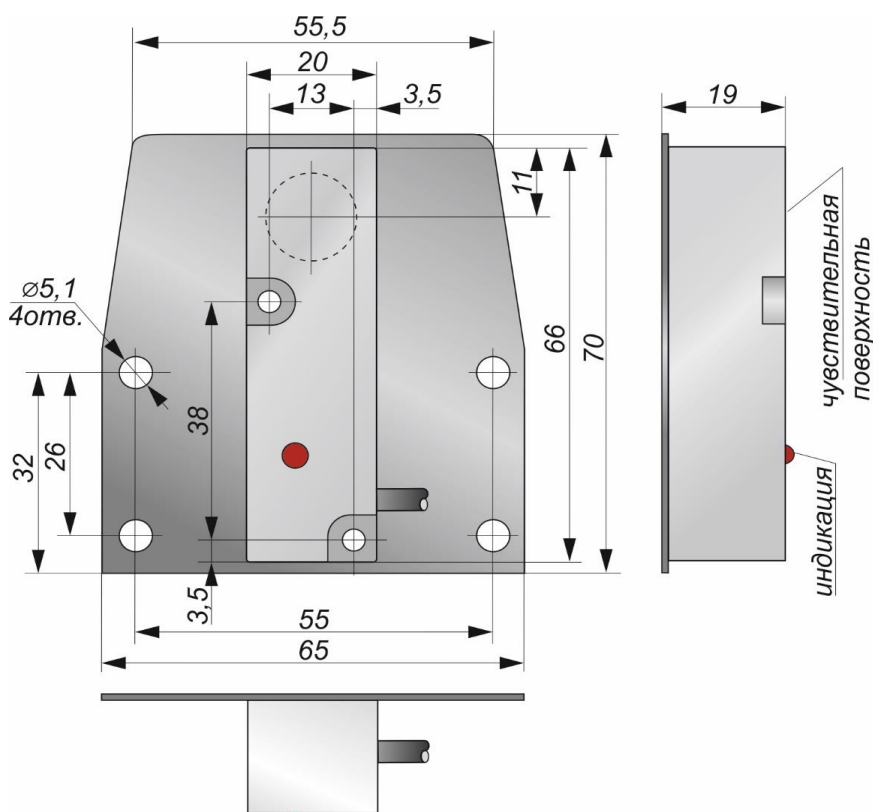
Габаритный чертеж
