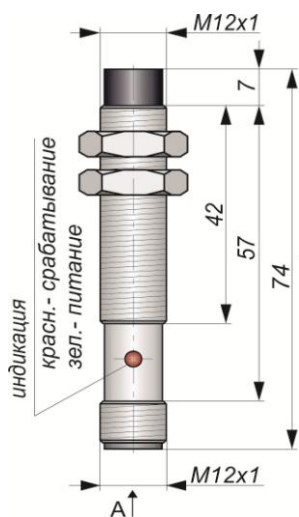
Габаритный чертеж
