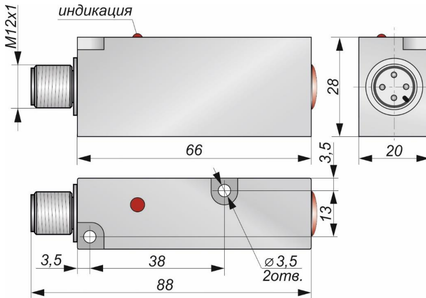
Габаритный чертеж
