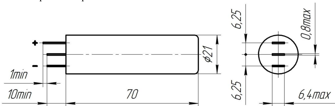
Нормально-замкнутый контакт
